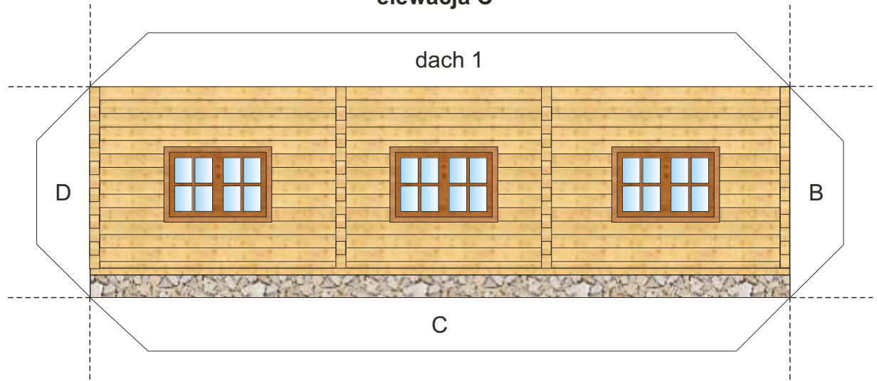
elewacja C
