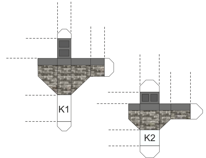
KOMIN K1, K2
