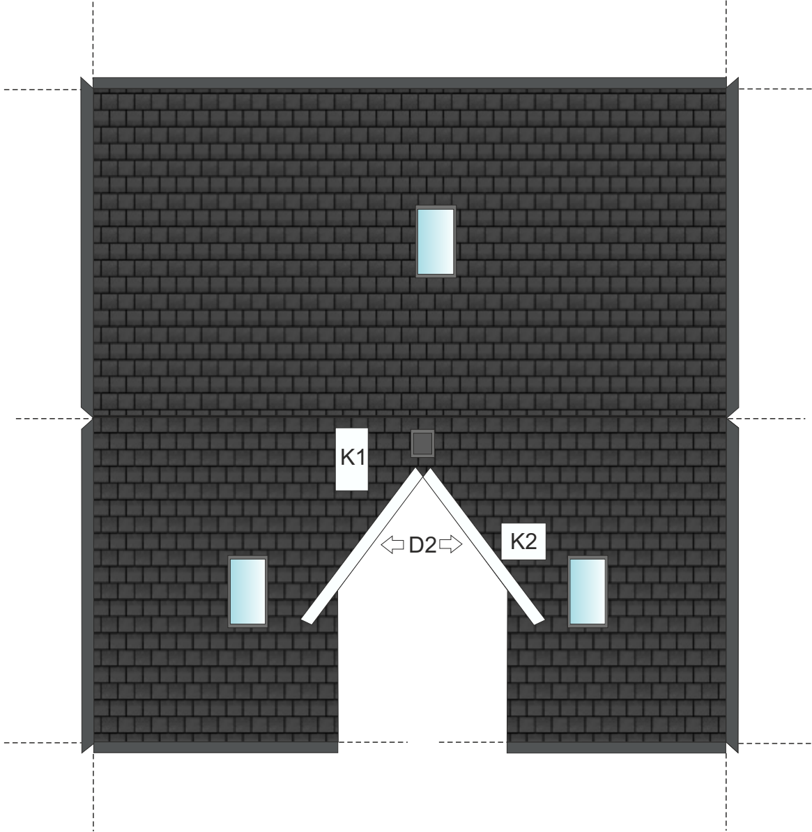
DACH D1
