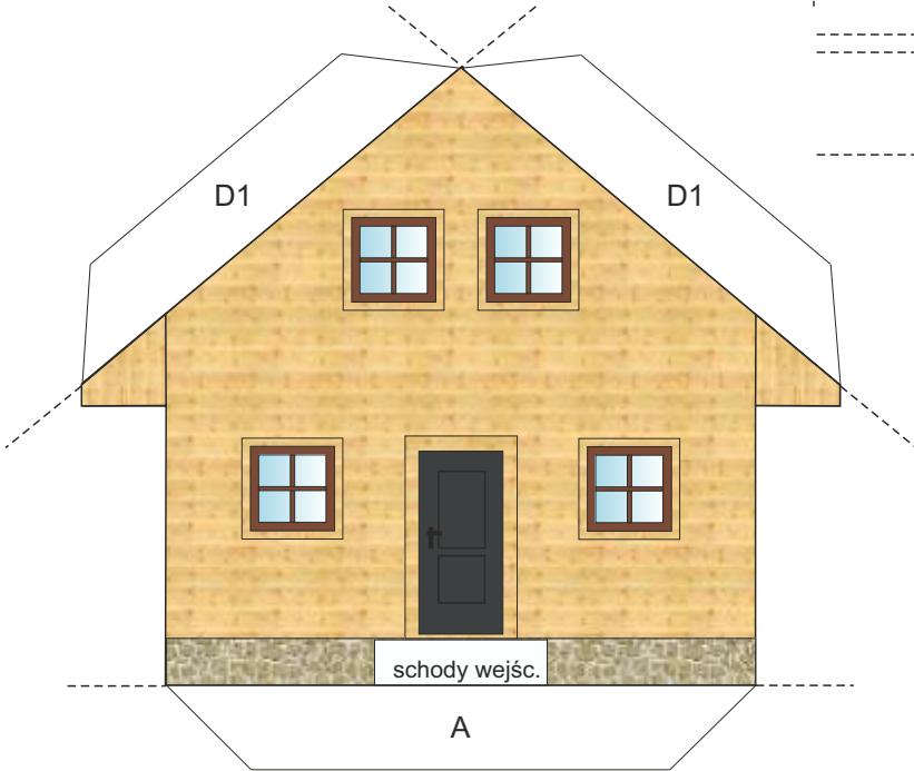
ELEWACJA A
