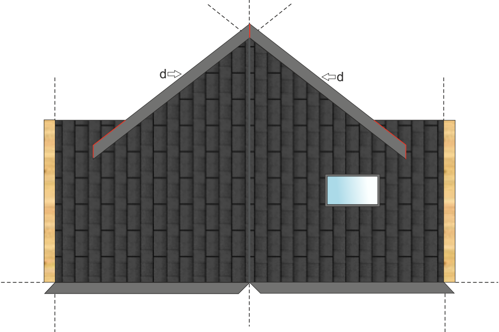
DACH D2
